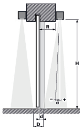
Sección transversal de la puerta corrediza, con sensores en ambos lados y campos de AIR opuestos
