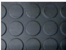
Struktura D Ø 23 mm, vzdálenost 25 mm výška výstupku 1,4 mm
